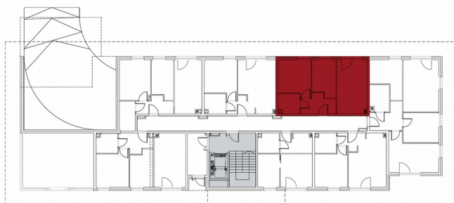
RZUT BUDYNKU B PARTER - LOKAL 4
