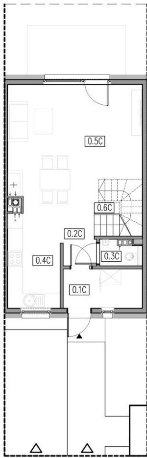
RZUT PARTERU
