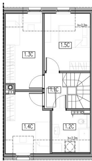
RZUT PIĘTRA
