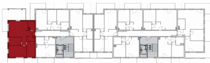
RZUT BUDYNKU C - KLATKA I 3 PIĘTRO- LOKAL 14
